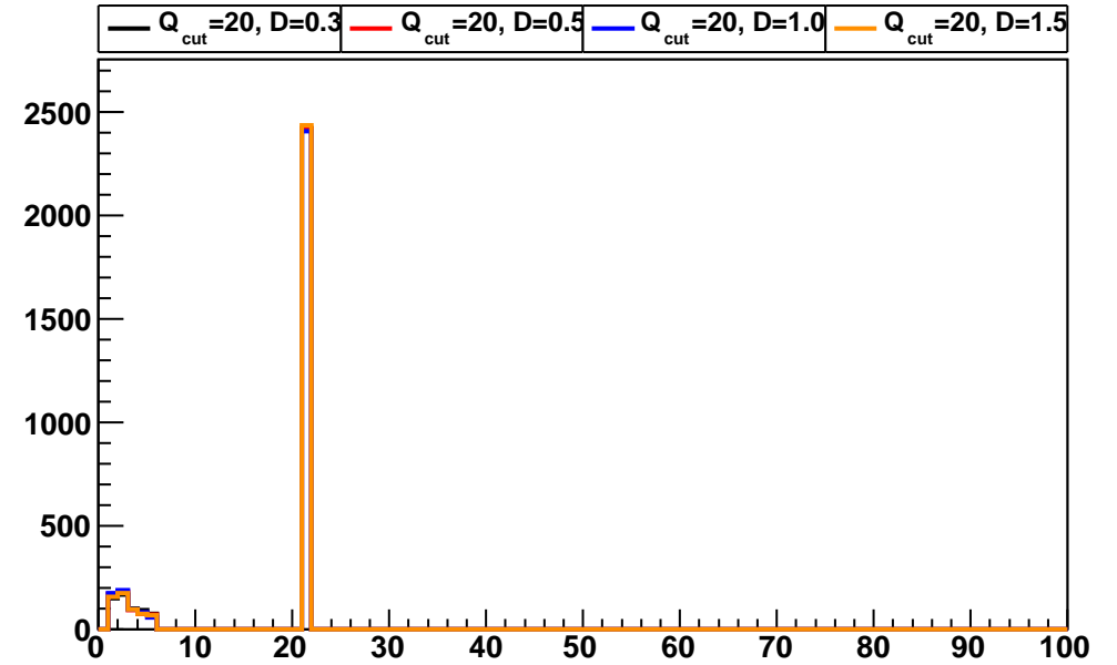
PDG id
